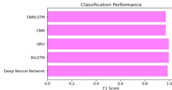
Fig 11 F1Score
